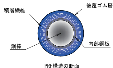
PRF 構造の断面
