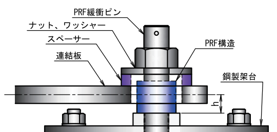
支点上構造高さが低い場合の構造
