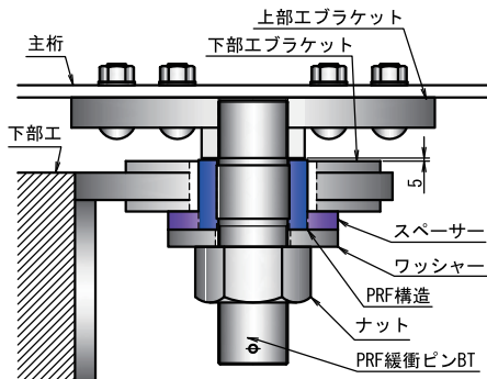
鉋桁に取付ける場合の構造
