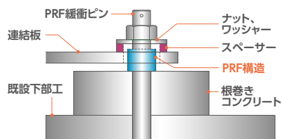
基本型（羽根連結－根巻コンクリート）
