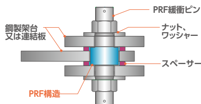
連結型（横断歩道橋、落橋防止）
