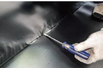
接合部チェック（ドライバー試験）
