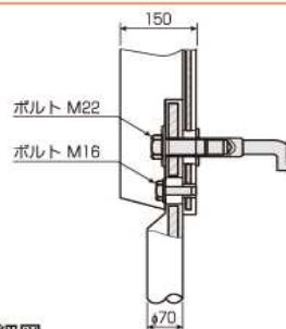
B部詳細図 150H型ラバータラップ+ジョイントラップ接続詳細図 (取付金具SVタイプ)
