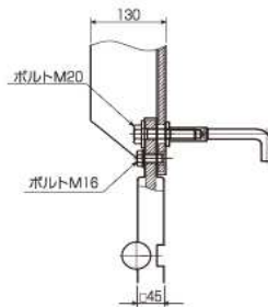
C部詳細図 130Hラバータラップ+ジョイントラップ接続詳細図 (取付金具SVタイプ)
