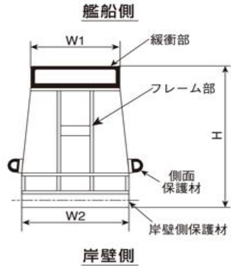
MF-S型（艦尾用）
